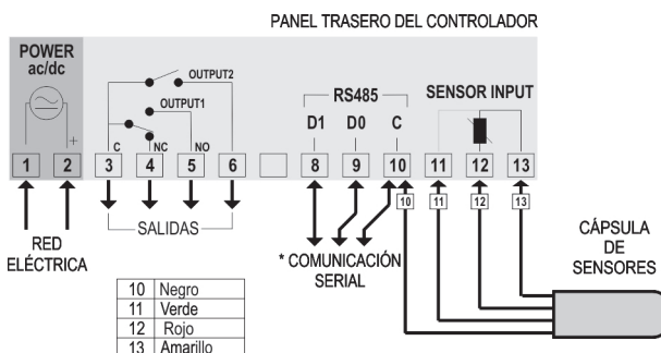
Fig. 2 - Conexiones mostradas en la etiqueta del controlador - Relés no aislados - Modelo Patrón
